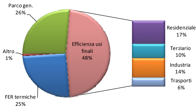
Ruolo dell'efficienza energetica nella riduzione delle emissioni di CO 2 nel 2020 nello Scenario Roadmap, rispetto allo Scenario di Riferimento per tipo di interventi (%)
