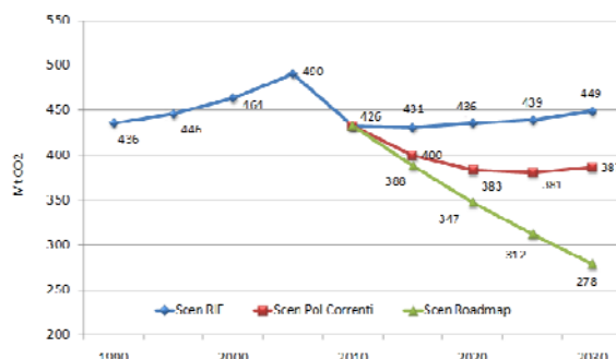
Evoluzione delle emissioni di CO 2 negli Scenari ENEA
