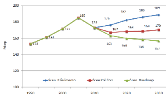
Evoluzione del fabbisogno di energia primaria
